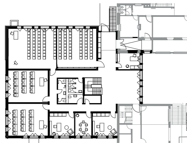
Grundriss Erdgeschoss
